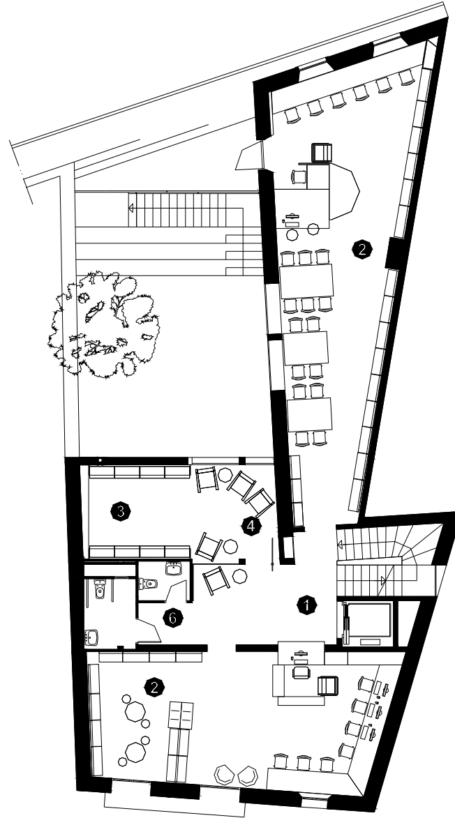
PLANTA PRIMERA
