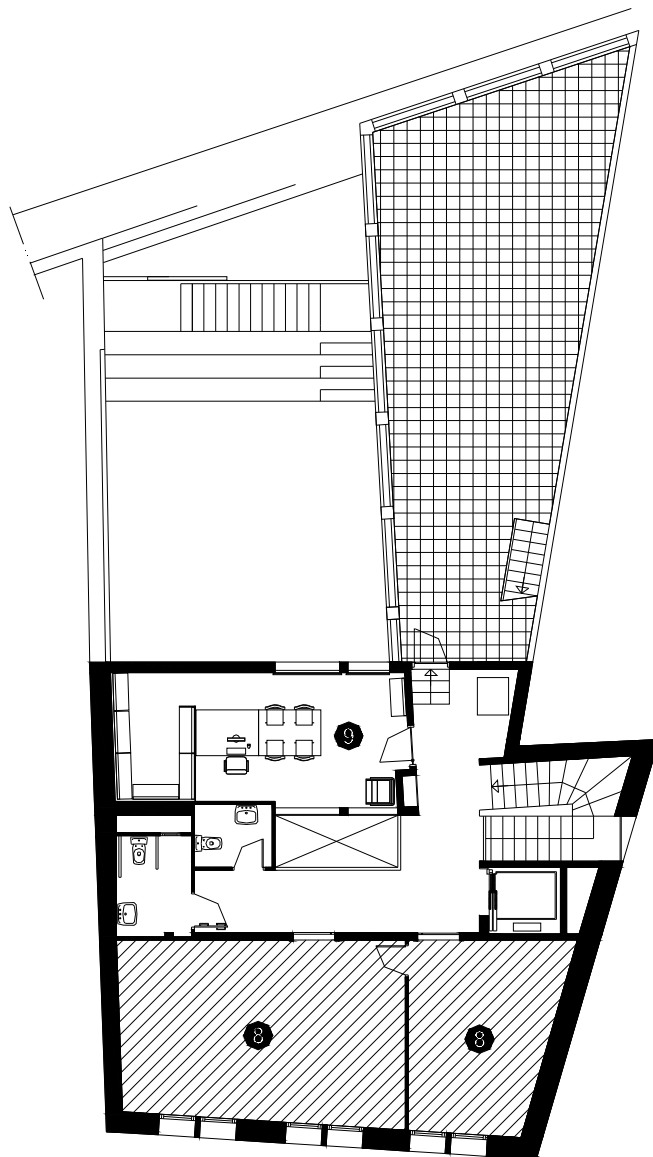
PLANTA SEGONA
