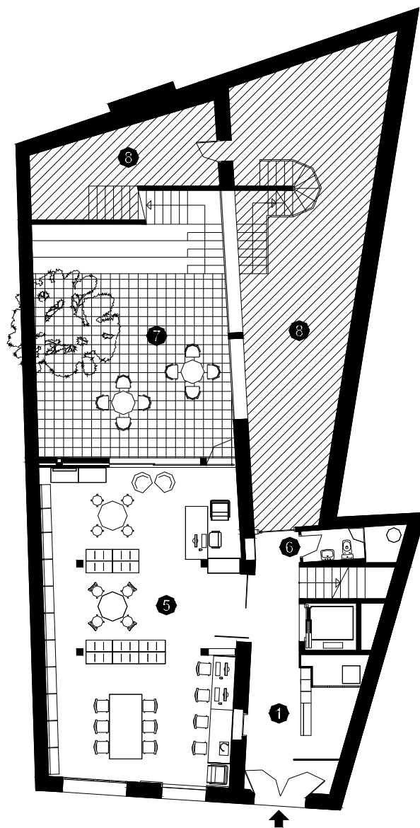
PLANTA BAIXA
