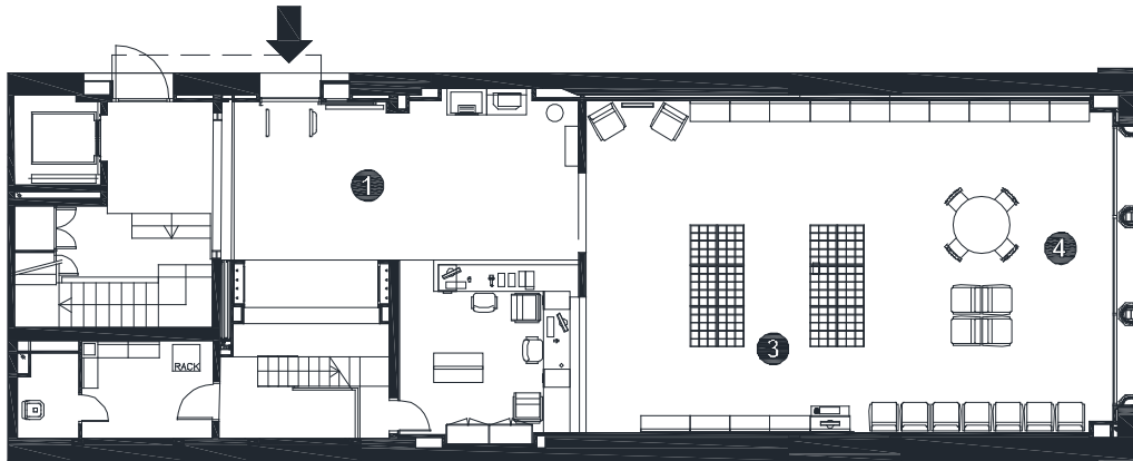
PLANTA BAIXA
