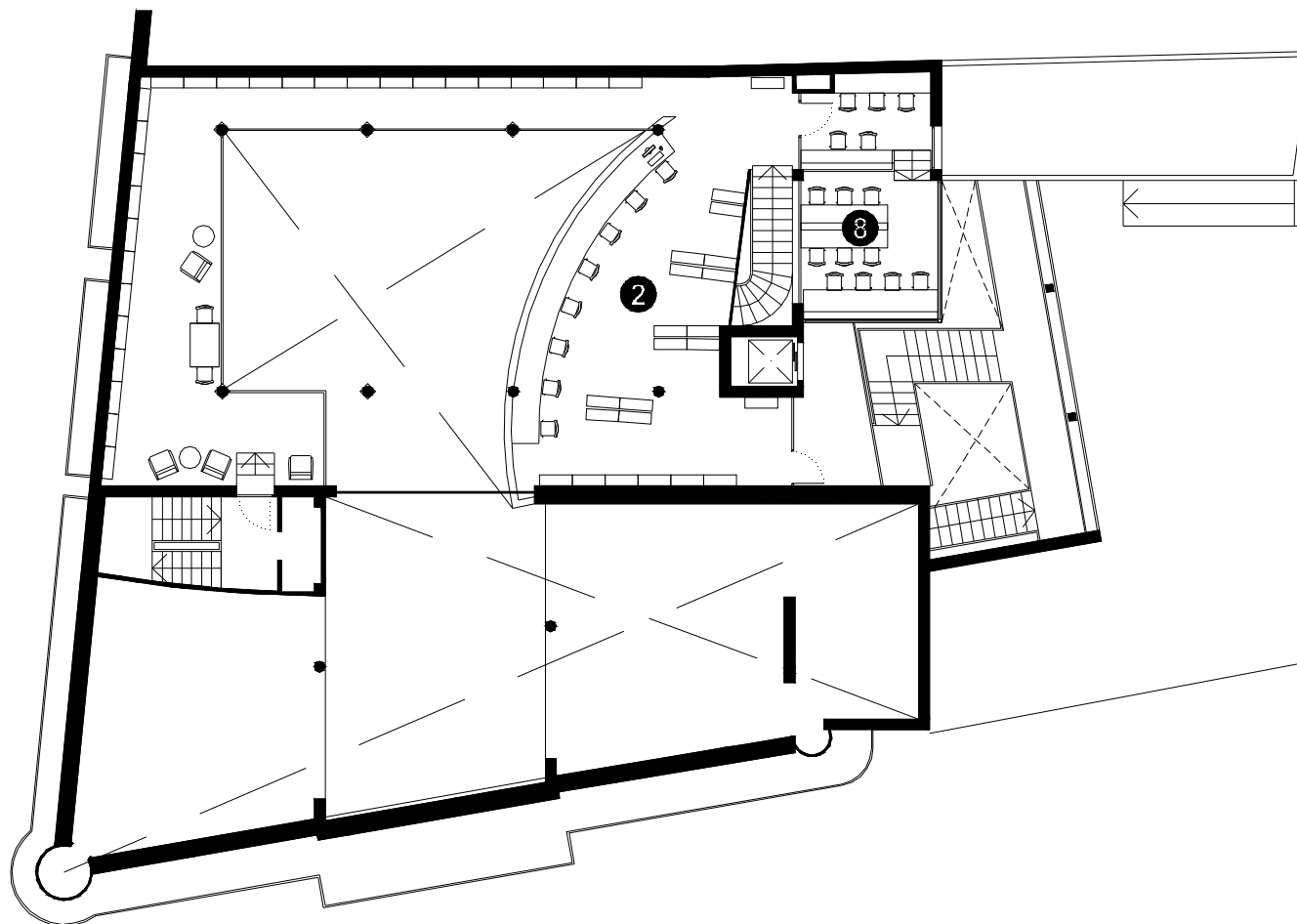
PLANTA SEGONA
