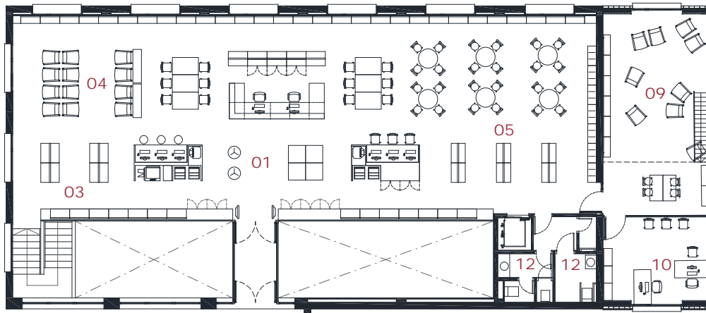
PLANTA ACCÉS
