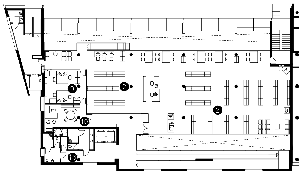
Planta Segona
