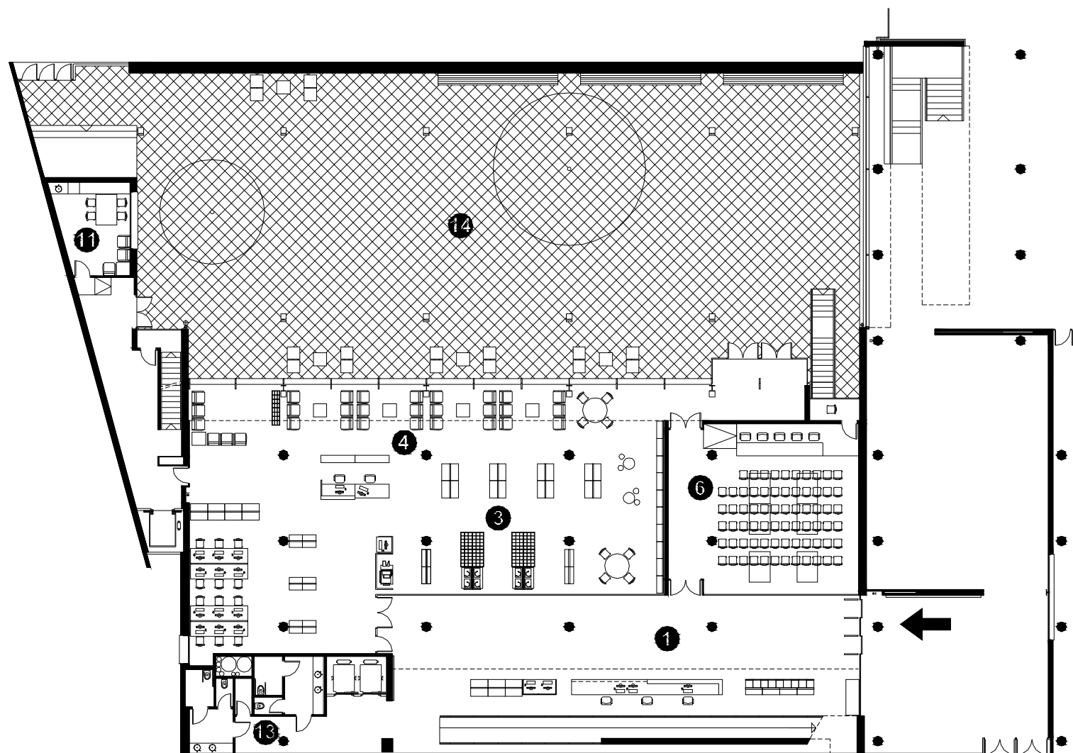
Planta Accés
