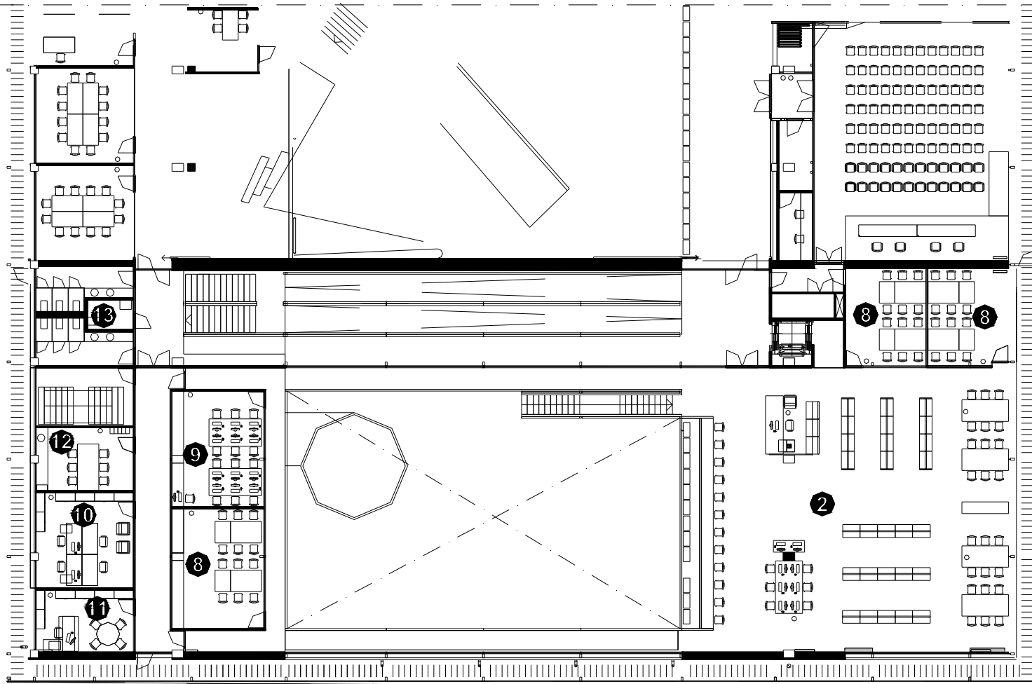
Planta superior
