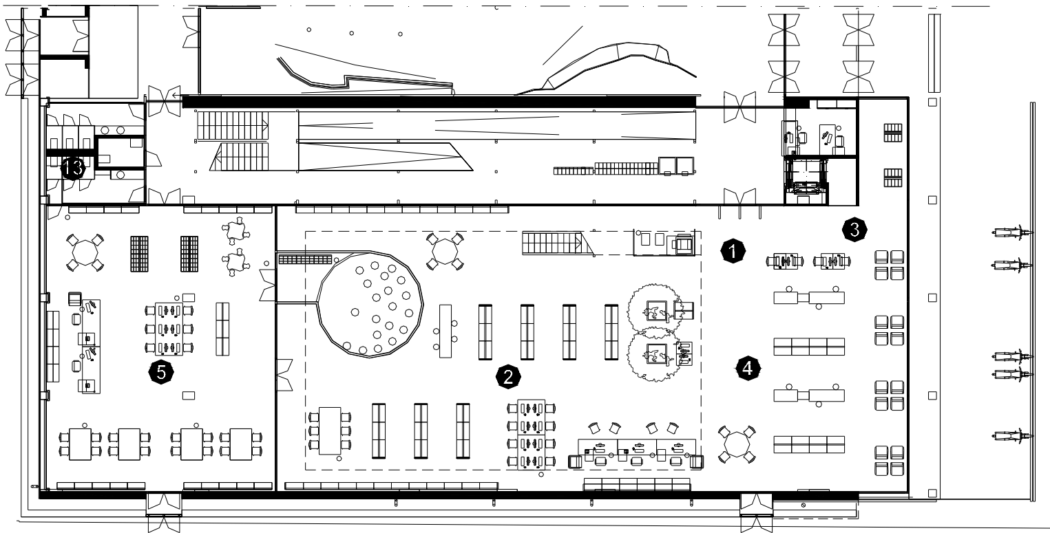
Planta accés
