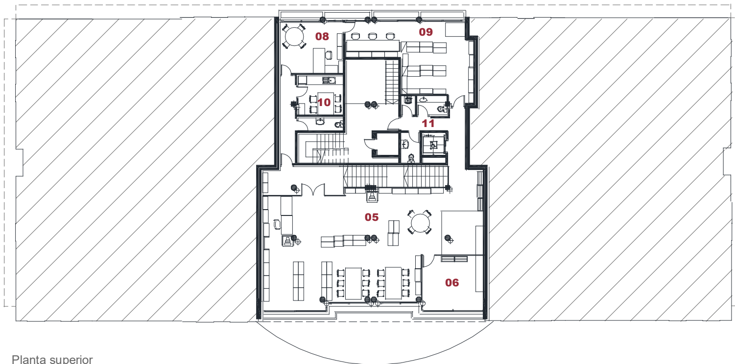
Planta superior
