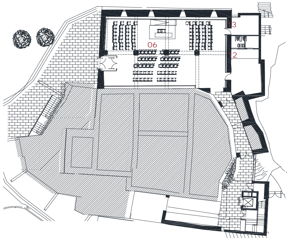
Planta inferior
