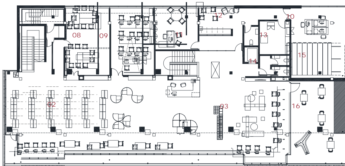
Planta superior
